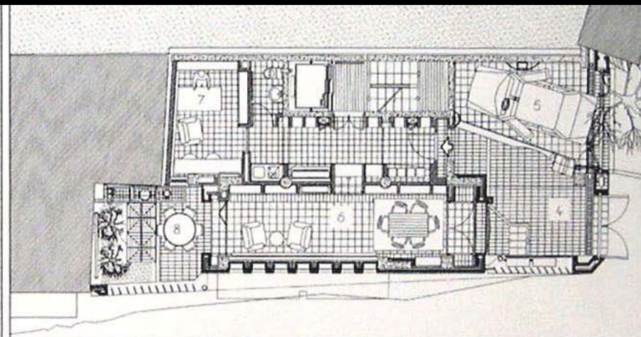
Κάτοψη Ισογείου
