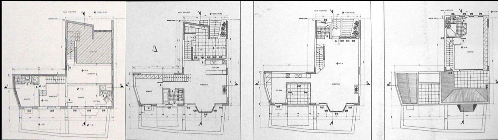
Κάτοψη α' - β' - γ' - δ' στάθμης και τομή κατά μήκος
